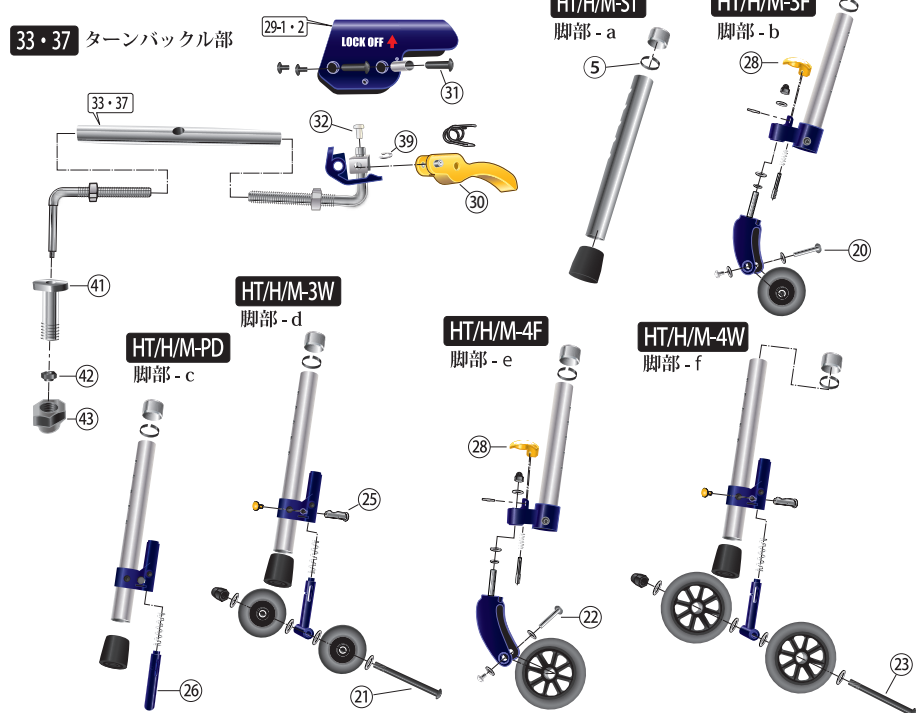
【各部のアッセンブリー図】
